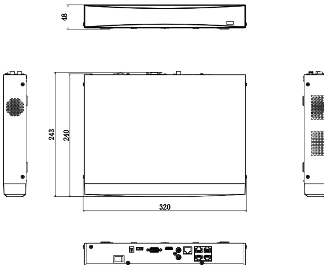
scale/1:1;Unit/mm
