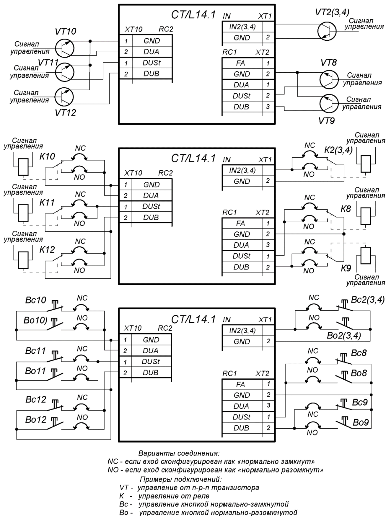
Рисунок 15. Схема подключений доп. оборудования к входам контроллера
