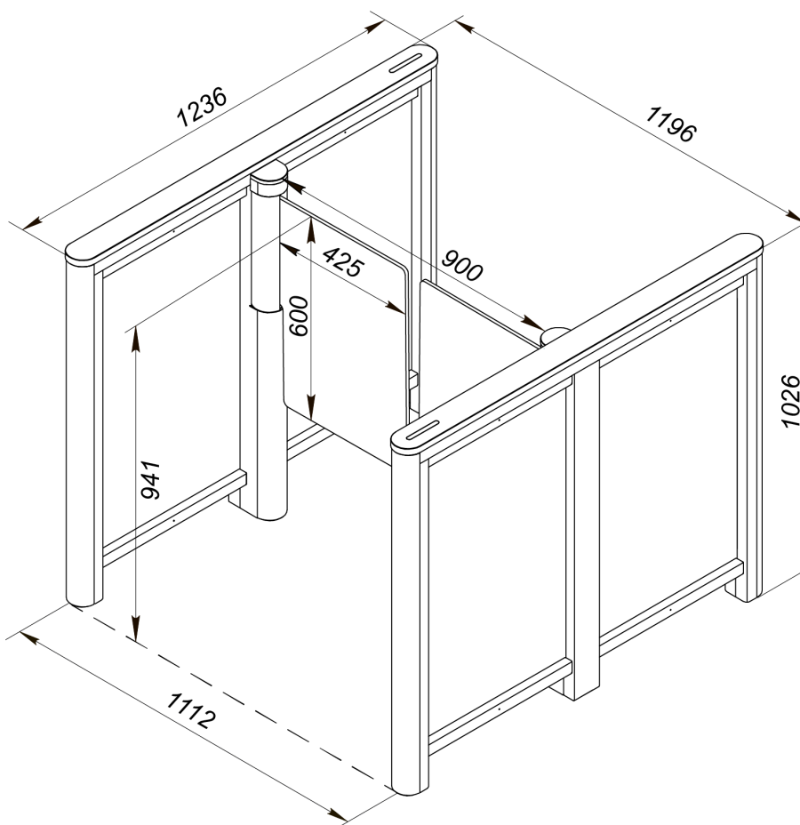
Рисунок 4. Габаритные размеры турникета со створками PERCo-ATG-475
