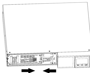
Шаг 2: Подключить провода аккумуляторных батарей
